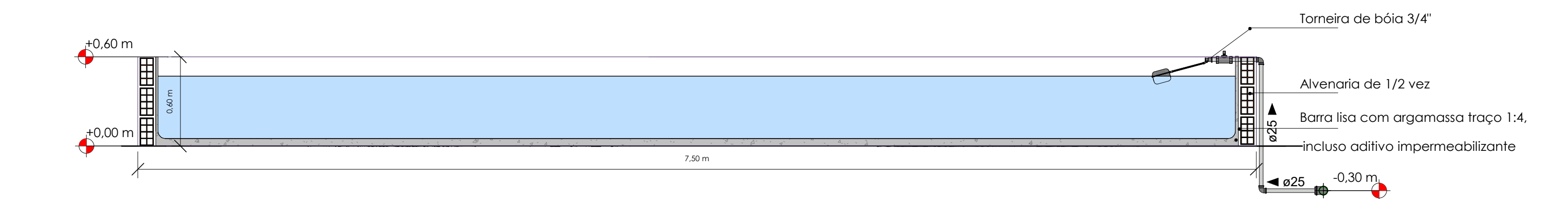
CORTE CC ESC 1/25
